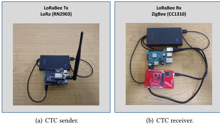
Fig. 4. Hardware.
